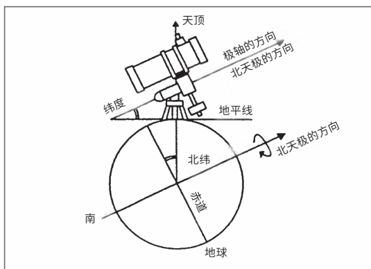
图 3-6 将赤道托架调整到地球的极轴方向
