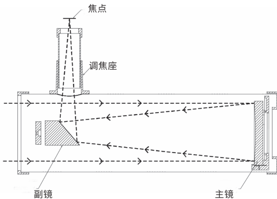
图 2-2 牛顿式反射望远镜光路剖面图
