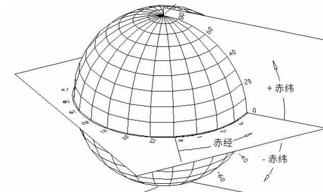
图 3-1 天球示意图
