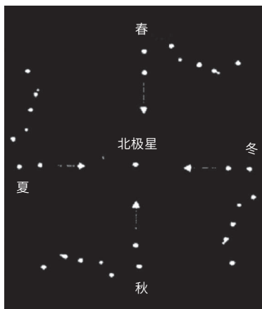
图 3-4 北斗七星在一年中的变化
