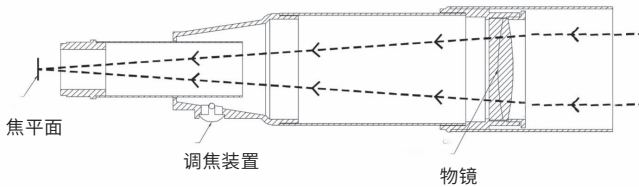
图 2-1 折射式望远镜光学设计的剖面光路
