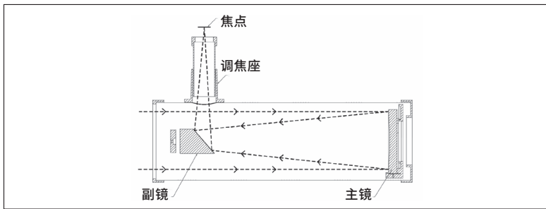
图 3-3 牛顿式反射望远镜光路剖面图
