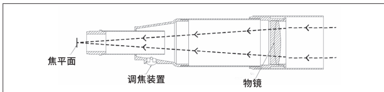
图 3-1 折射式望远镜光学设计的剖面光路
