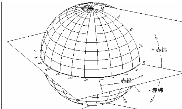
图 4-1 天球示意图
